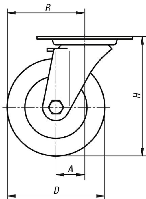
Kormányzott görgő
