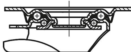
Forgócsapágyazás: csavaros lemez
