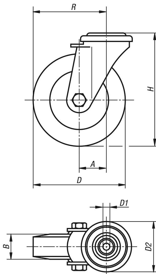
Forgócsapágyazás:
