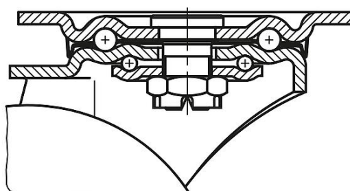
Forgócsapályazás R1-től = 160
