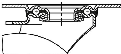
Forgócsapályazás R1-ig = 125
