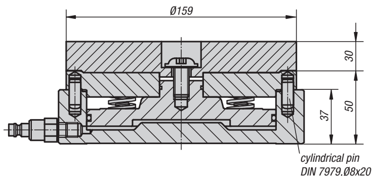
view A-A
