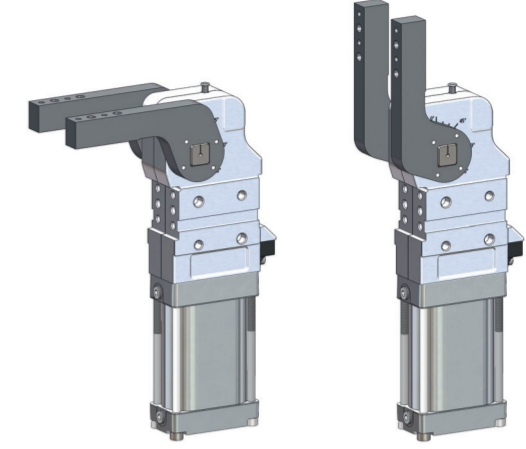
82M-3E23... Arm links/rechts 90° 82M-3E23... Arm links/rechts 180°
