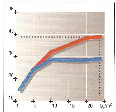
Egyrétegű térelválasztó elem hanggátlása a felületre vonatkoztatott tömeg függvényében. A piros vonal a kimondottan kis hajlítózsilárdságra vonatkozik.
