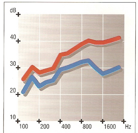
Kék vonal: Közönséges forgácslap hanggátlási görbéje. Piros vonal: HAWAPHON-nal a teljes felületen összeragasztott forgácslap hanggátlása.
