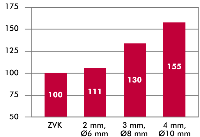
Druckluftverbrauch je Zyklus [%]
