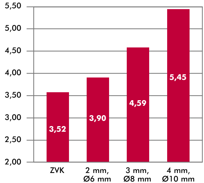
Druckluftverbrauch je Zyklus [l]
