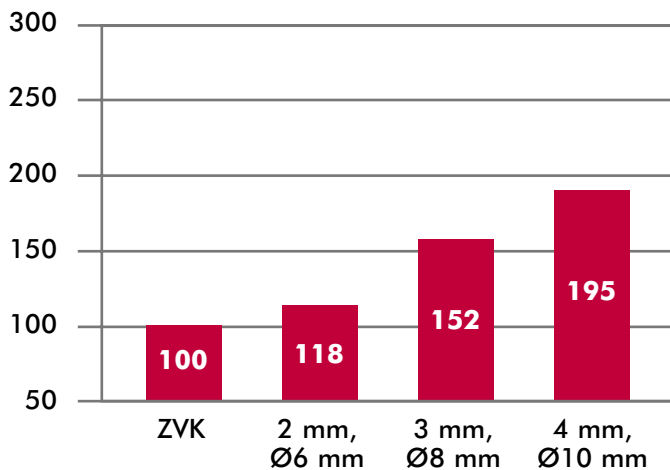
Druckluftverbrauch je Zyklus [%]
