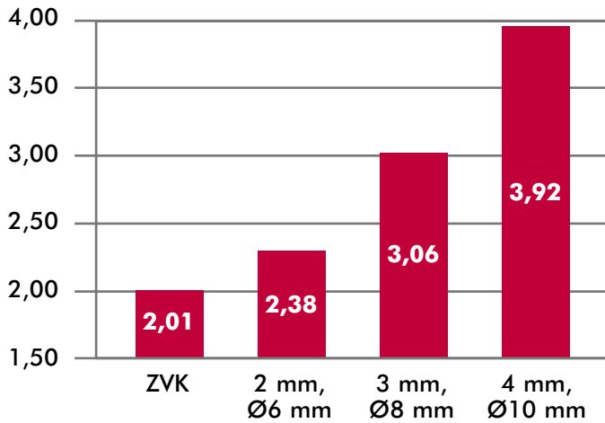
Druckluftverbrauch je Zyklus [l]
