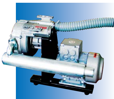
Vakuumberläse mit Keilriemenantrieb und Abluftschalldämpfer.
