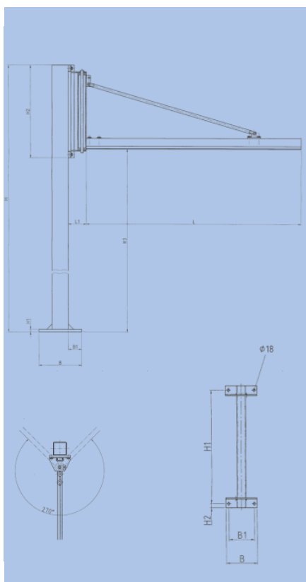
Säulenschwenkkrane SSK 125-4.000 für Lasten bis 60 kg
