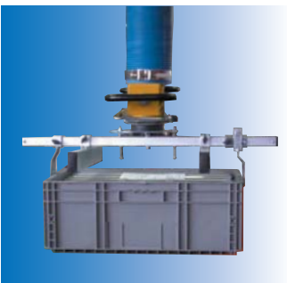
VacuPowerlift VPL mit mechanischem Spezial-Saugfuß für das Handling von Transportkisten
